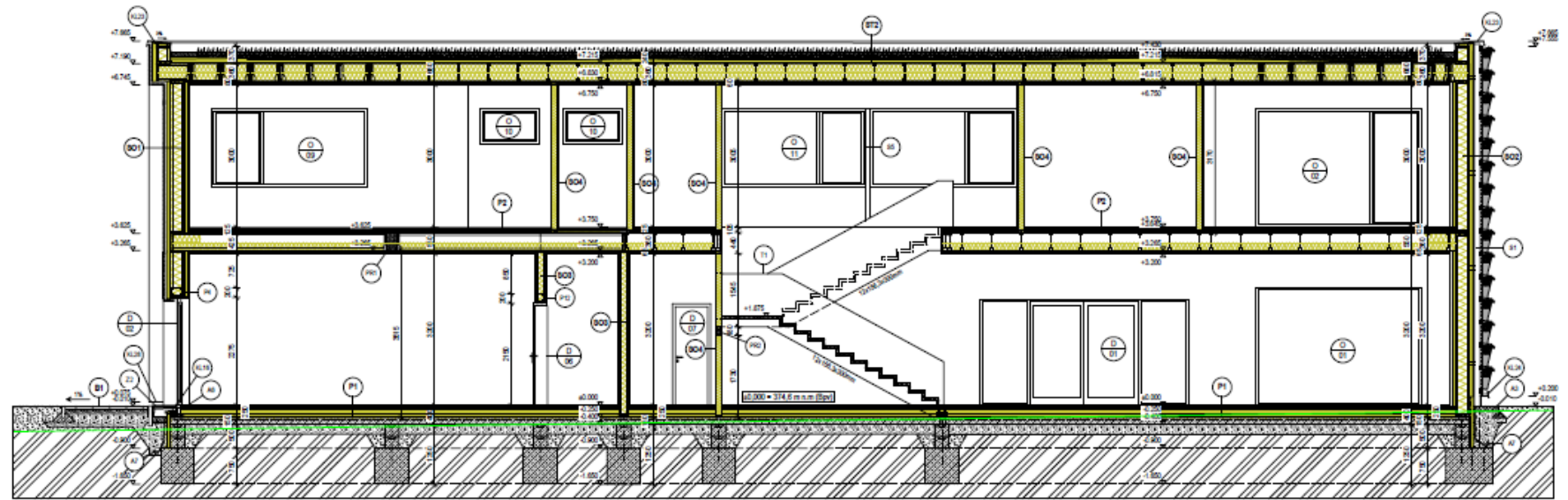
ŘEZ A - A
