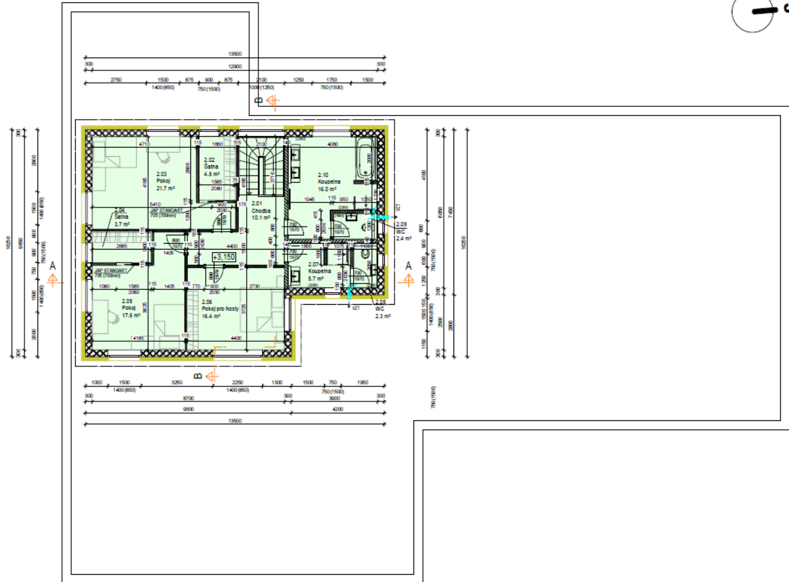
PŮDORYS 2.NP
