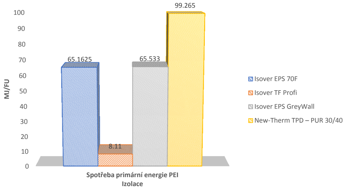
Porovnání PEI
