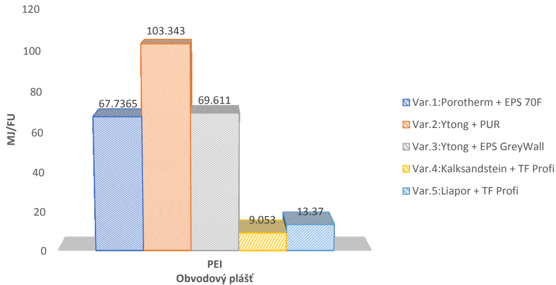
Porovnání PEI
