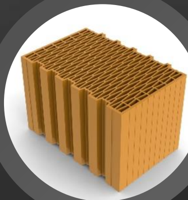
Keramické tvárnice
