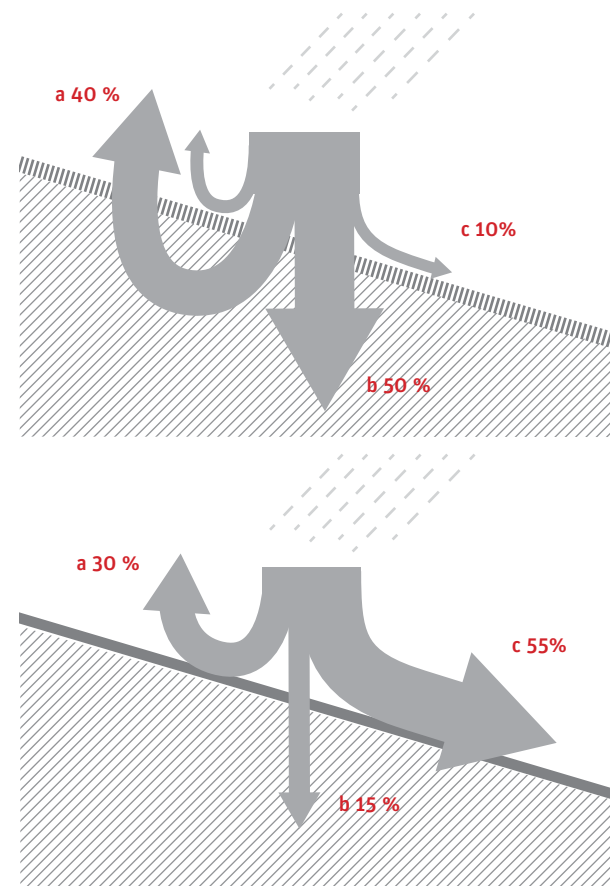
s21 ROZDÍL V PODÍLU POVRCHOVÉHO ODTOKU NA KRAJINNÝCH A ZPEVNĚNÝCH PLOCHÁCH
