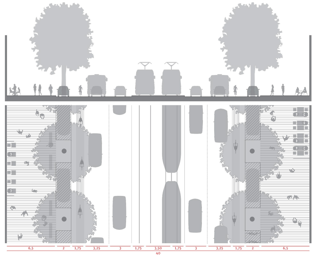
s14 MĚSTSKÁ OSA (ŠÍŘKA 40 M)
